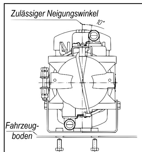
Abb. 3 - Befestigung des FLOW 14D
