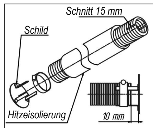
Abb. 13 – Auspuffschild
