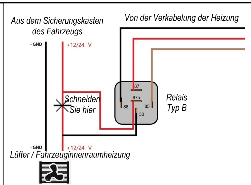
Abb. 27 – Anschlussdiagramm für FLOW 5
