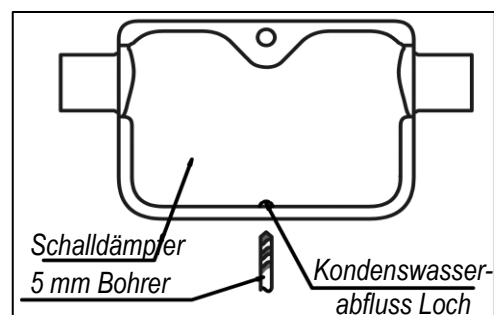
Abb. 14a – Kondenswasserabflussloch für horizontale Befestigung
