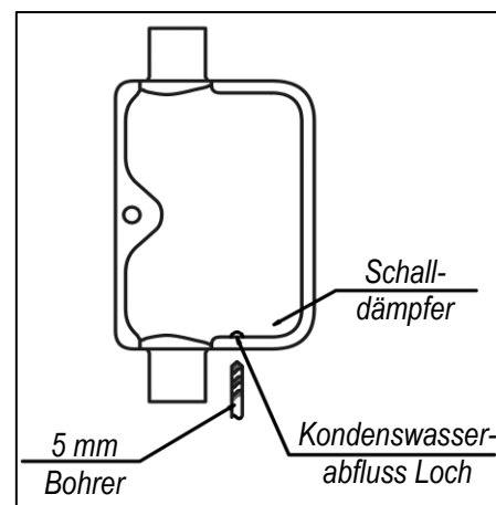
Abb. 14b – Kondenswasserabflussloch für vertikale Befestigung
