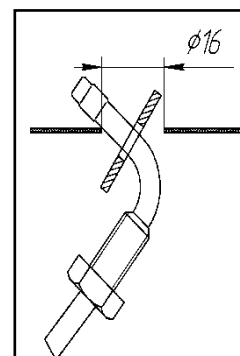
Abb. 19b – Installation der Unterlegscheibe
