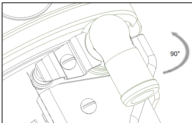
Abb. 6b – Winkelleitungsbefestigung für FLOW 14D
