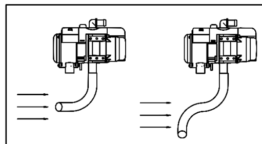
Abb. 8 – Position des Lufteinlassrohres/Auspuffs
