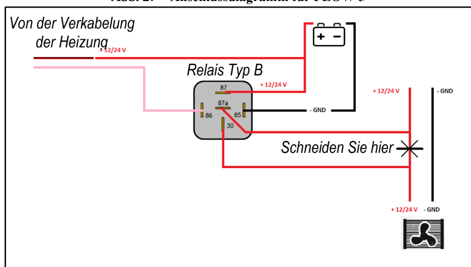
Abb. 28 – Anschlussdiagramm für FLOW 14D
