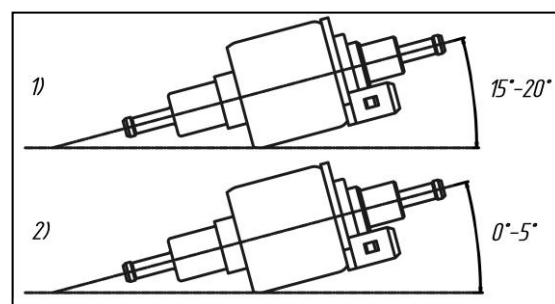
Abb. 22 – Installationswinkel der TH-9; TH-10; TH-11-Kraftstoffpumpe (1) und Thomas Magnete-Kraftstoffpumpe (2).
