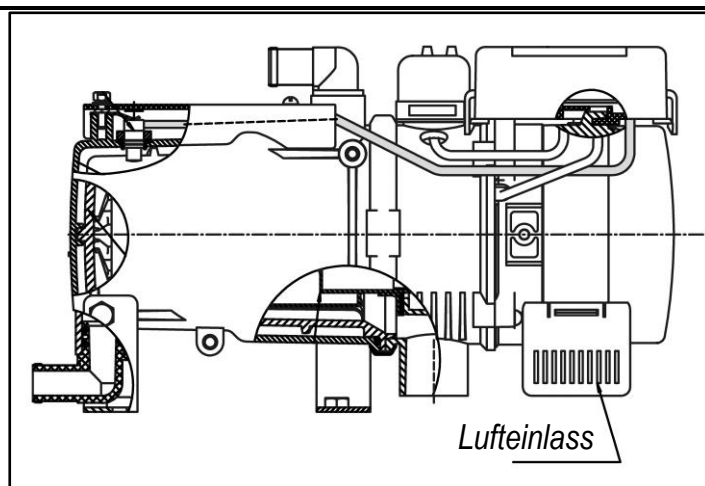
Abb. 7b – Lufteinlass des FLOW 14D
