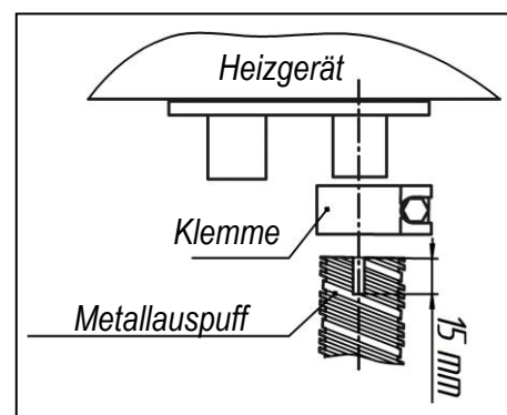
Abb. 11 - Anbringung des Metallschlauchs an das Heizgerät
